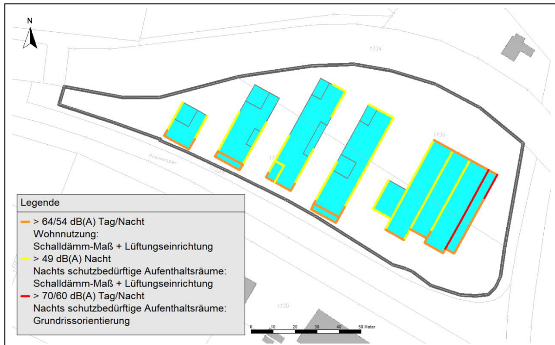
Abbildung 11: Verkehrslärm – Erforderliche Schallschutzmaßnahmen Baukörper (Wohnen)
